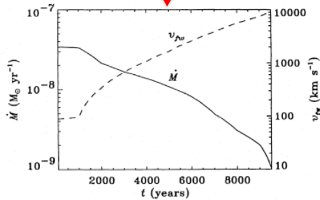
Mellema (1994, A&A, 290, 915)
